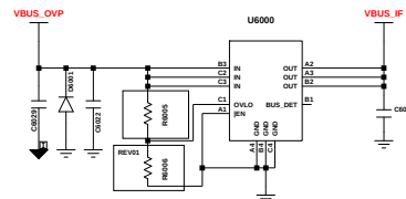
OVP
